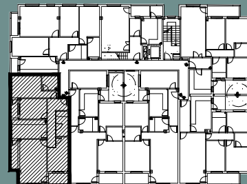
PLANTA ESQUEMA
